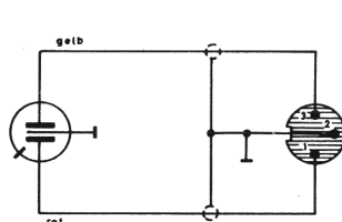
Stechverbindung zwischen Laufwerk und Chassis
